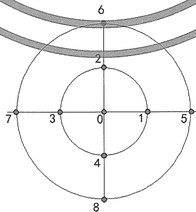
图1 色温与显色指数测试模板测点示意图
