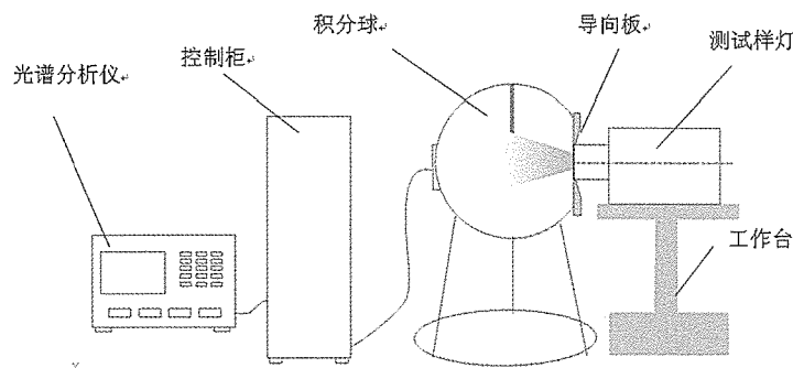
图2 积分球法测量示意图
